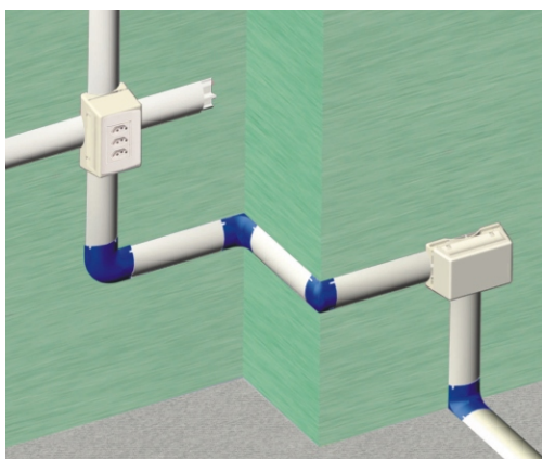
Exemplo de instalação com duto slim.
